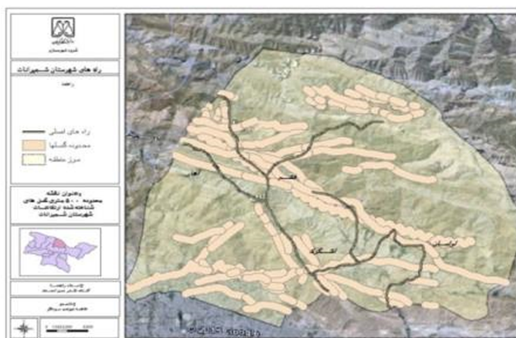
شکل ۷- وضعیت گسل‌های منطقه و بافر ۱۰۰۰ متری در اطراف آن.
