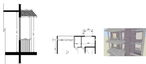
الف: نمای مدل پایه تحقیق در حالت سایه اندازی با ایوان
