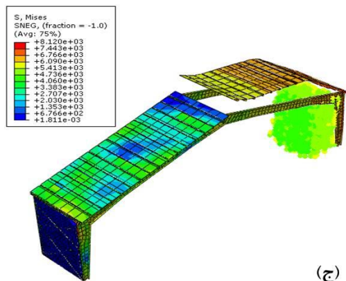
شکل ۳: تغییر شکل سازه پس از انفجار. الف) ۷٫۵ کیلوگرم معادل TNT ماده منفجره، ب) ۲۵ کیلوگرم معادل TNT ماده منفجره، ج) ۳۵ کیلوگرم معادل TNT ماده منفجره، د) ۵۰ کیلوگرم معادل TNT ماده منفجره؛ در فاصله ۱۰ متری بیرون سازه (نگارندگان)
