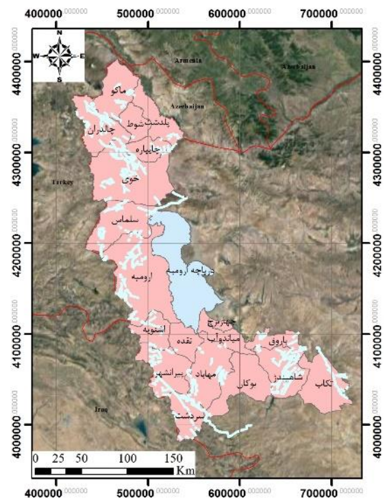
نقشه ۲. گسل‌های موجود در استان آذربایجان غربی
