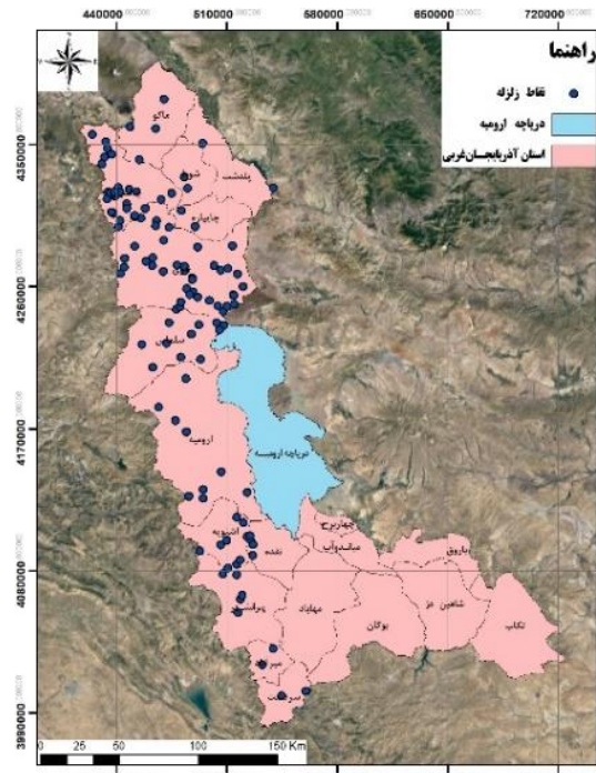
نقشه ۳. داده‌های نقطه‌ای زلزله‌های صورت گرفته طی سال‌های ۱۳۰۹-۱۳۹۷
